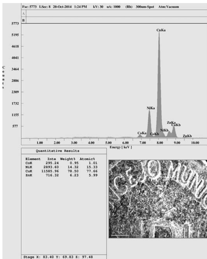
Fig. 4. Anàlisi d'una moneda d'1 pta. (niquelada) amb microfluorescència de rajos X (μFRX).
